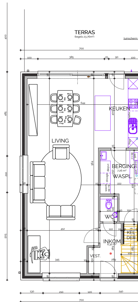
Gelijkvloers
