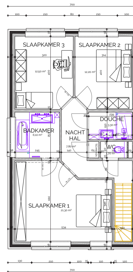
Verdieping
